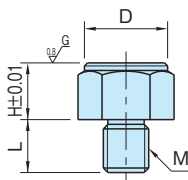
BJ811-F (先端研磨タイプ)
