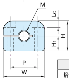
AMBH (水平固定型)
