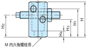
BJ210 (标准型)
