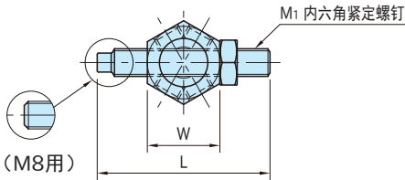
(标准型)
