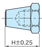
BJ810-S (前端锯齿型)
