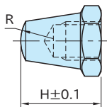
BJ810-R (前端R型)
