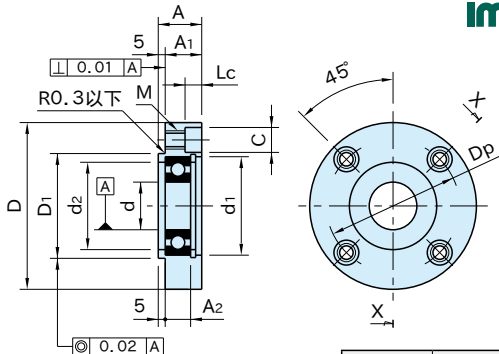
剖面 X-X
