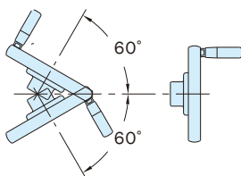
显示器安装时的角度范围
