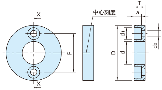
剖面 X-X
