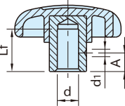
EK-R EK-R-SUS (高精度孔)
