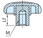
EK-T EK-T-SUS (内螺纹孔)
