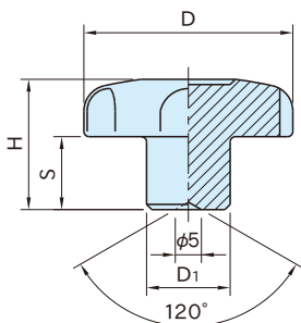
(无孔)
