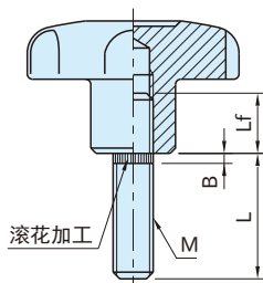
(外螺纹)
