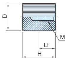
LKN-SUS (内螺纹孔)
