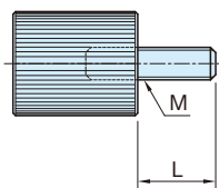
LKS-SUS 5~10 (外螺纹)
