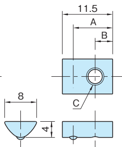
L5-TST-SUS (ステンレススチール製)
