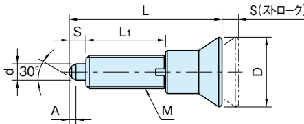
SDXN SDXN-SUS SDXN-A-SUS (ナット無し)
